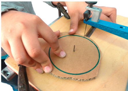
Abb. 156 | Sägehilfe für Räder (Bezug www.do-it-werkstatt.ch )
