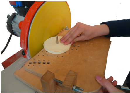
Abb. 155 | Schleifhilfe für Räder, geeignet für Holz- und Kunststoffräder aller Dicken (Bezug www.do-it-werkstatt.ch )
