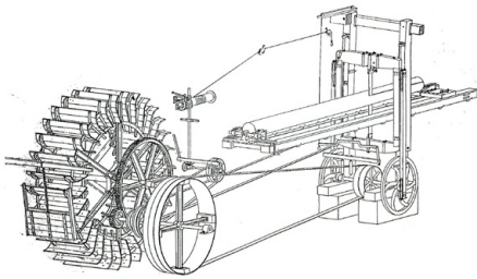
Abb. 222 | Säge mit Mühlradantrieb
