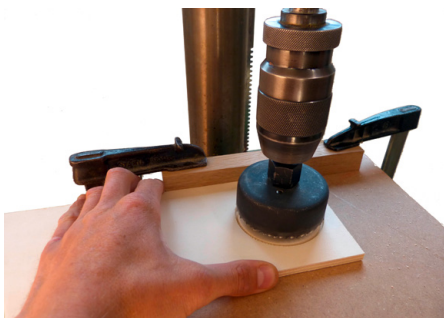
Abb. 157 | Glockensäge nur mit Anschlag benutzen.
