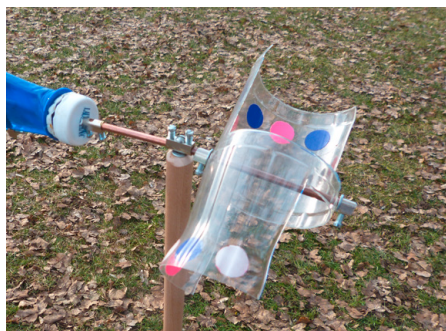
Abb. 290 | Rohrwindrad
