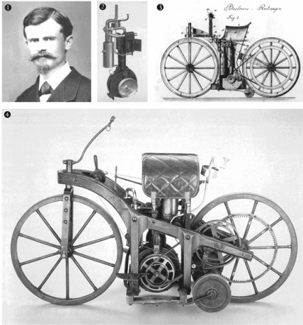
Abb. 121 | Wilhelm Maybachs Petroleum-Reitwagen
