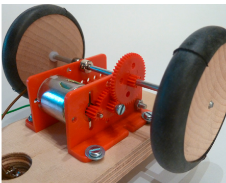
Abb. 187 | Bausatz Getriebemotor
