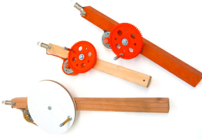
Abb. 255 | Dynamotaschenlampe
