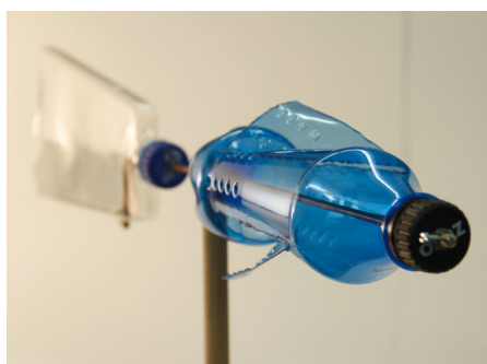
Abb. 289 | Raketenwindrad
