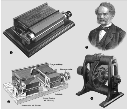
Abb. 136 | Werner von Siemens' Dynamomaschine
