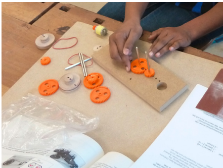
Abb. 147 | Kinder experimentieren in der Lernwerkstatt Getriebeversuche.
