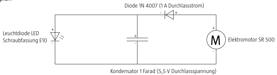
Schaltplan
