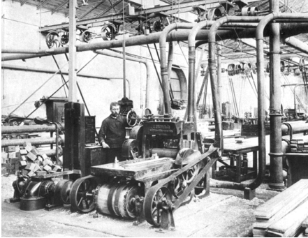
Abb. 135 | Fabrikhalle mit elektrischem Einzelantrieb und Transmissionsriemen
