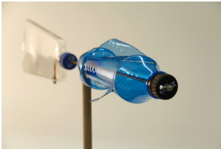
Abb. 270 | Raketenwindrad
