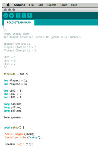
Abb. 292 | Sketch in der IDE
