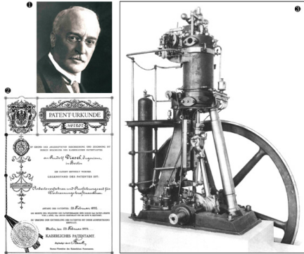
Abb. 117 | Rudolf Diesel und sein Motor
