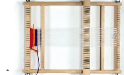
Tischwebrahmen: Rahmen mit Kettbaum, Warenbaum, Gatterkamm und Schiffchen.
