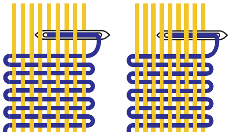
Grundbindungen: Je nach Verlauf des Schussfadens entstehen unterschiedliche Webbindungen.
