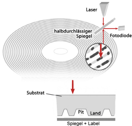
Abb. 153 | Auslesevorgang bei einer CD. Das Licht trifft auf die Pits und Lands und wird entsprechend reflektiert.
