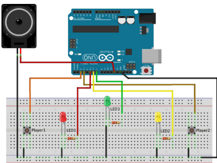
Abb. 167 | Schaltplan von «Ready-Steady-Baam» in der Steckplattenansicht
