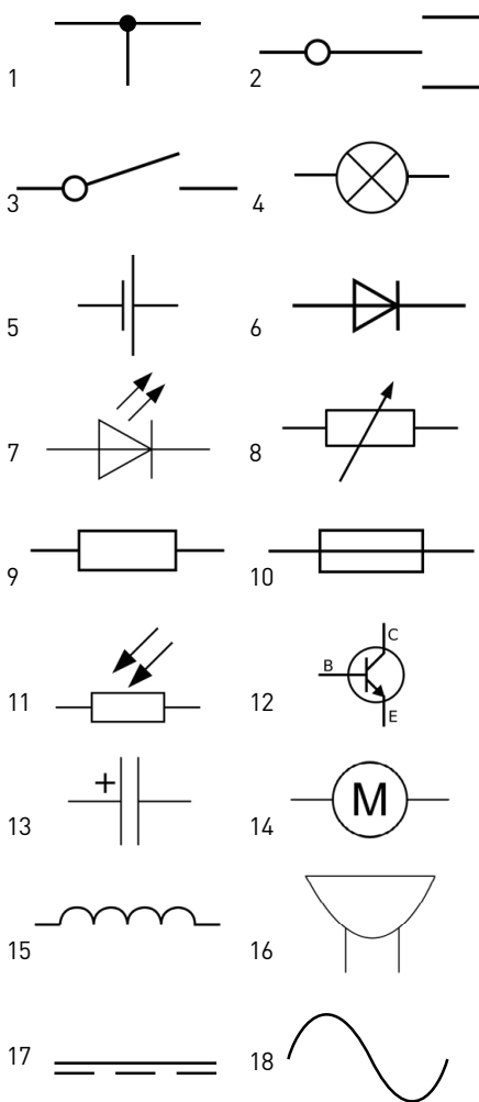
Abb. 133 | Schaltsymbole: 1: Leiter mit Verzweigung, 2: Umpolschalter, 3: Schalter, 4: Glühlampe, 5: Batterie, 6: Diode, 7: Leuchtdiode (LED), 8: Potenziometer, 9: Widerstand, 10: Sicherung, 11: Fotowiderstand, 12: Transistor, 13: Elko (gepolter Kondensator), 14: Motor, 15: Spule, 16: Summer, 17: Gleichstrom, 18: Wechselstrom
