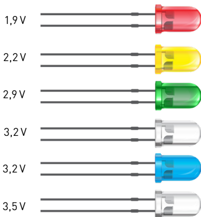
Abb. 134 | Durchlassspannung verschiedener LEDs
