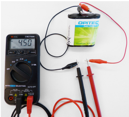
Abb. 135 | Spannungsmessung an einer 4,5-V-Batterie
