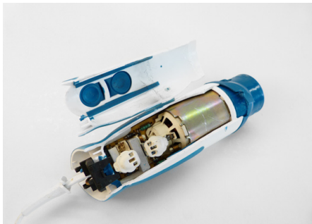
Abb. 131 | Elektromotor eines Küchenmixers
