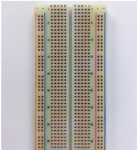
Abb. 168 | Steckplatine mit eingezeichneter Linie zum Stromfluss
