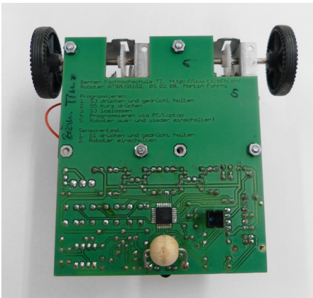
Abb. 160 | Der Microcontroller als Gehirn eines Roboters
