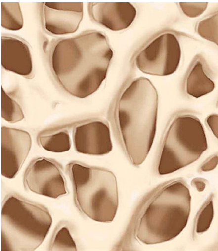
Abb. 121 | Das Prinzip der Knochenstruktur lässt sich auf die Technik übertragen. Stark belastete Stellen werden verstärkt, an weniger belasteten Stellen wird Material entfernt.
