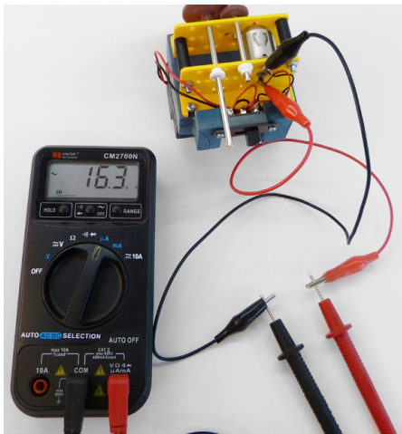
Abb. 136 | Strommessung an einem Getriebemotor
