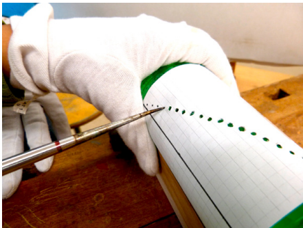
Abb. 276 | PET-Flasche mithilfe der Schablone und der erhitzten Ahle perforieren.
