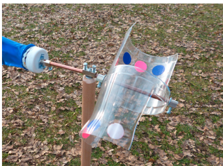
Abb. 290 | Rohrwindrad
