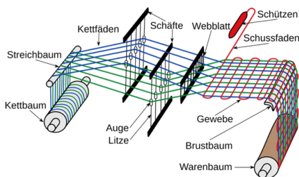
Abb. 64 | Prinzip einer Webmaschine mit zwei Schäften
