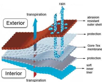
Abb. 56 | Aufbau von Goretex Textilien
