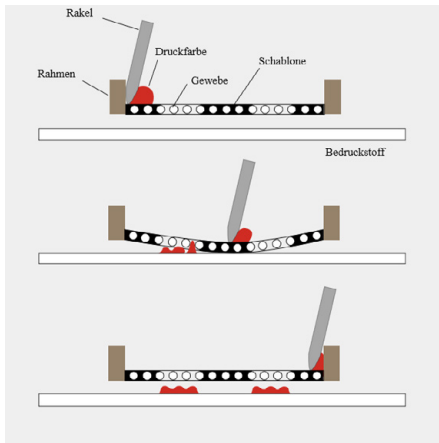
Abb. 78 | Schema des Siebdruckverfahrens
